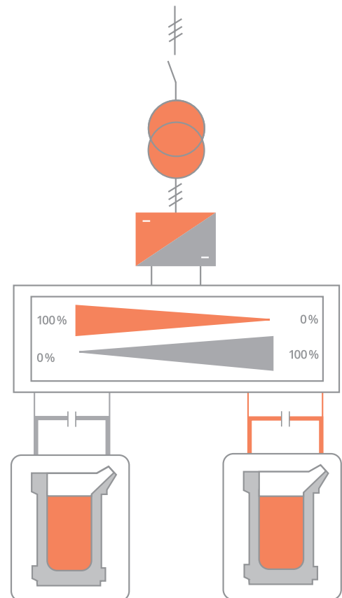
TWIN-POWER® Prinzip
